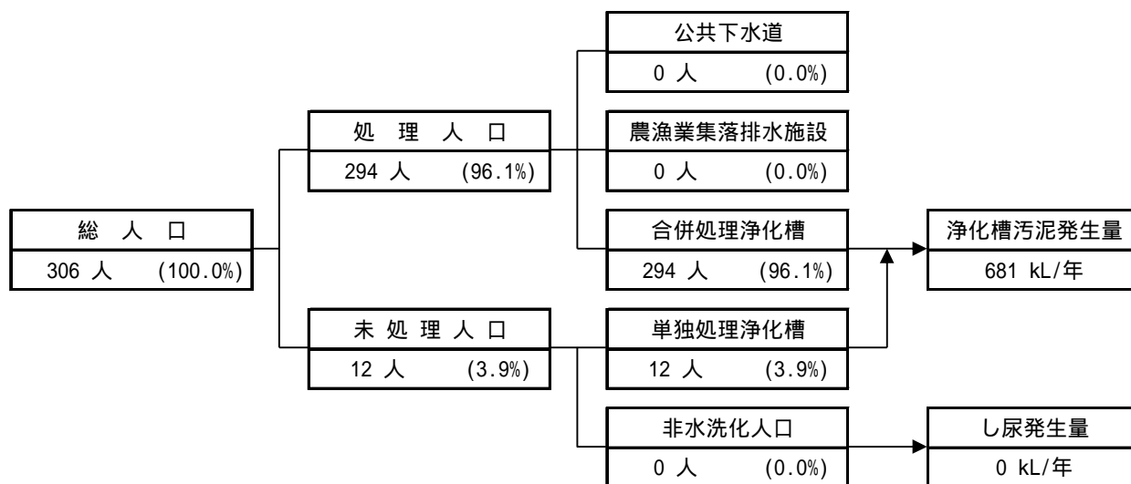
図2 生活排水処理の処理状況フロー（平成27年度実績）
