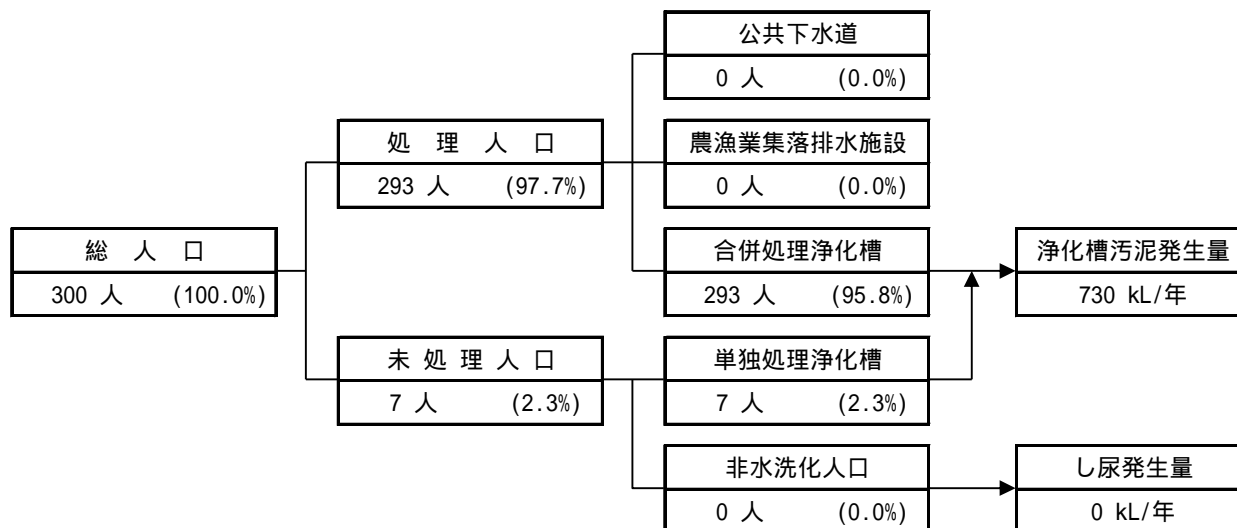
図3 生活排水処理の処理状況フロー（平成34年度目標）
